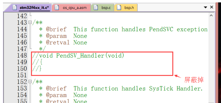
图 4.3.3.2 屏蔽函数
