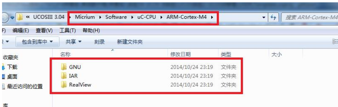
图 4.2.3 ARM-Cortex-M4 文件夹
