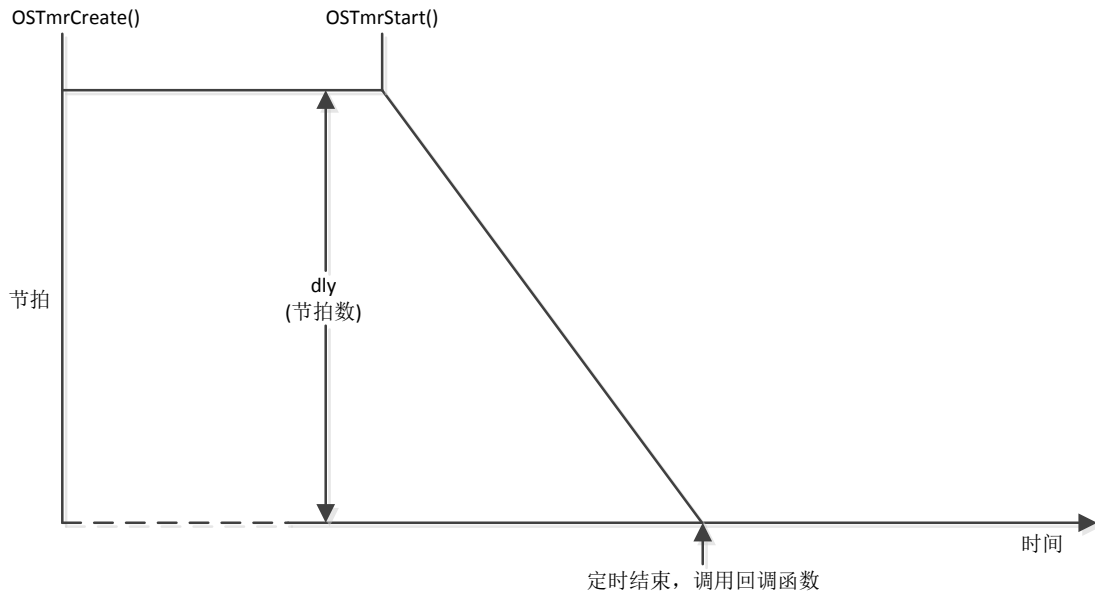
图 9.1.1 单次定时器
