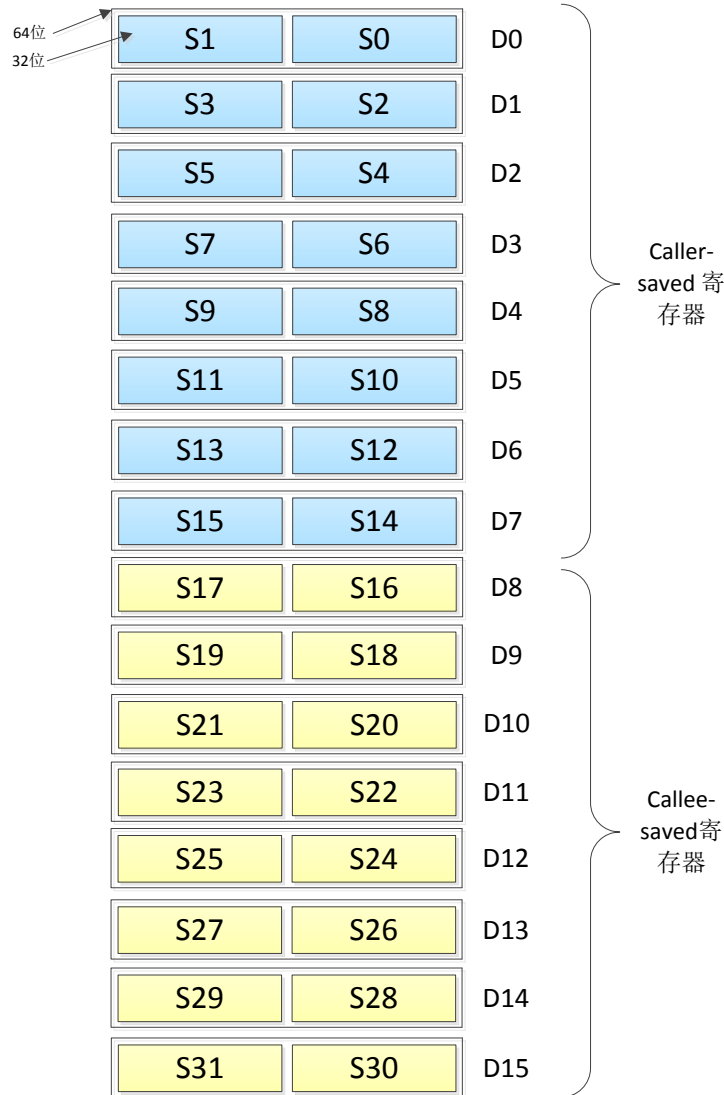
图 2.3.1 浮点寄存块
